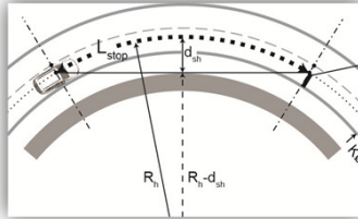
Stopsigt ved lang kurve
