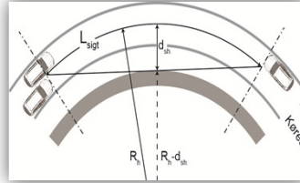
Mødesigt og overhalingssigt, lang kurve
