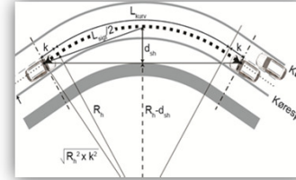
Stop-, møde- og overhalingssigt, kort kurve
