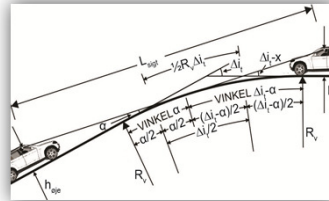
Stop-, møde- og overhalingssigt, kort konveks kurve
