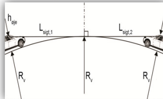
Stop-, møde- og overhalingssigt, lang konveks kurve
