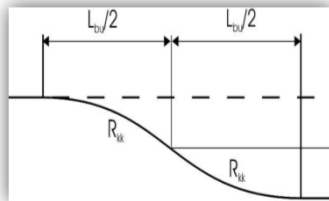
Breddeudvidelse, lige vej
