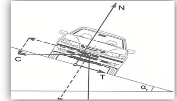
Tværfald og radius med kørselsdynamik
