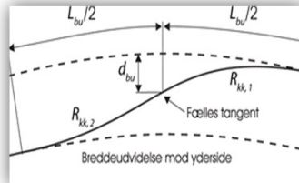
Breddeudvidelse, kurvet vej
