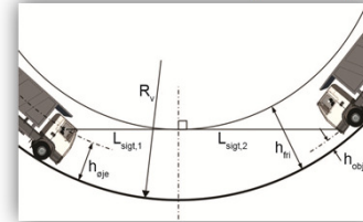
Stop-, møde- og overhalingssigt, konkav kurve ved sigthindring
