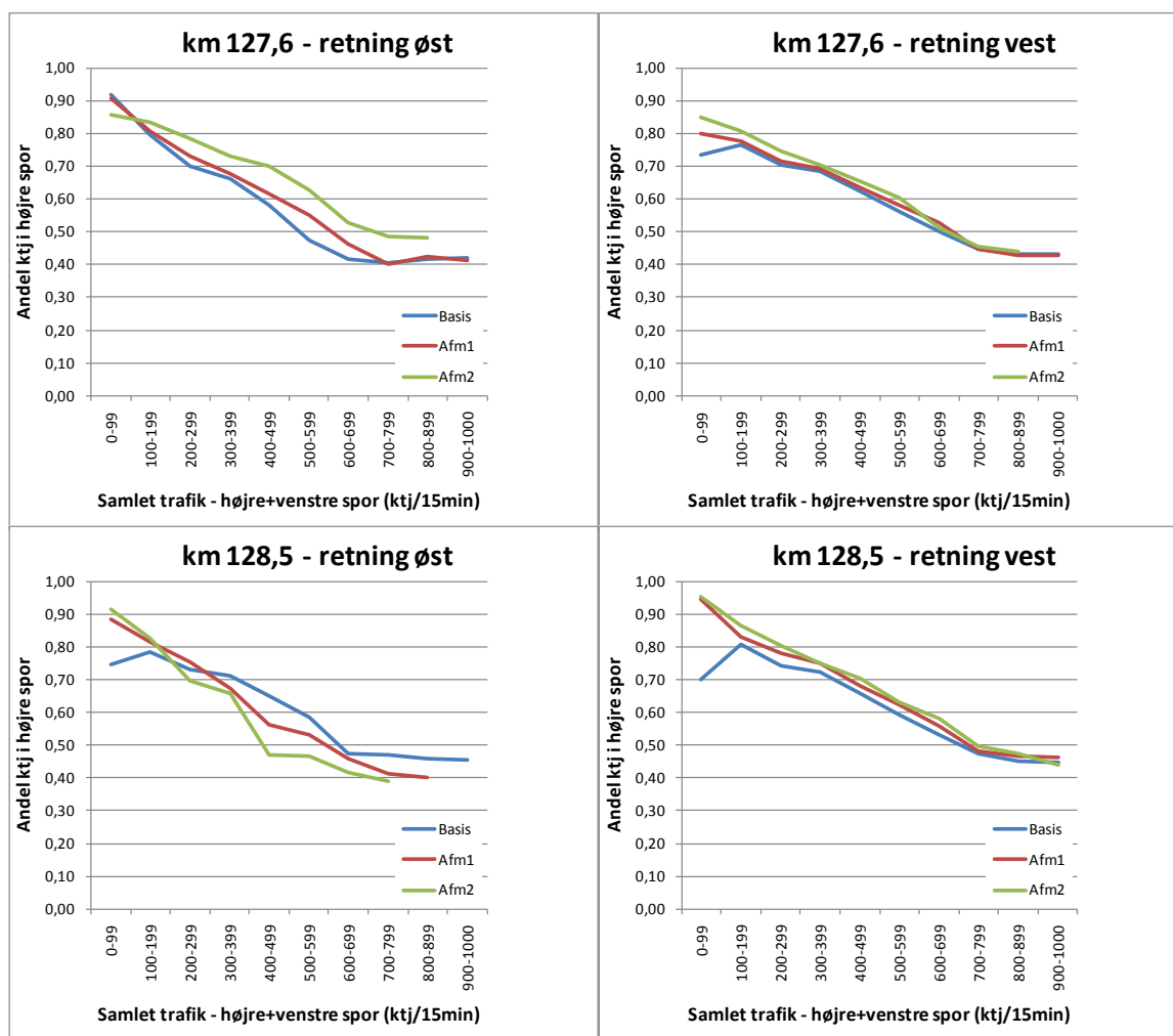
Figur 3.7. Andel køretøjer i højre kørespor som funktion af den samlede trafik.
