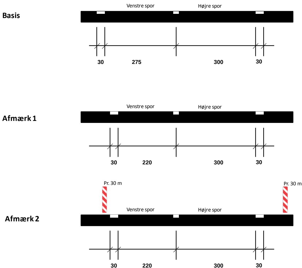
Figur 2.2. Sporbredde og placering af N42 (kantplade) ved de tre opstillinger.
