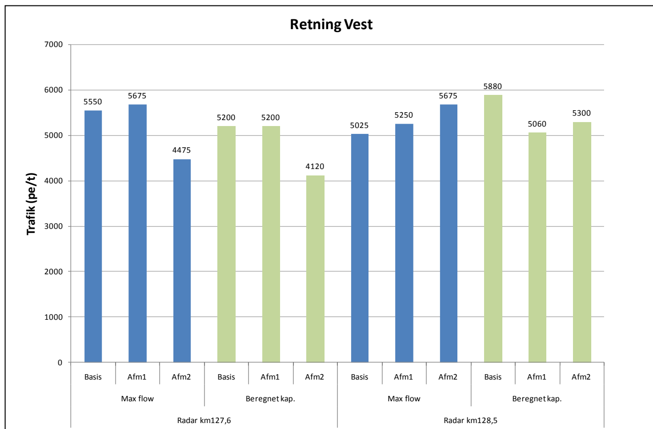
Figur 3.5. Observeret maksimal gennemstrømning og beregnet kapacitet for retning vest. (beregnet kapacitet for km 128,6 er usikkert bestemt)
