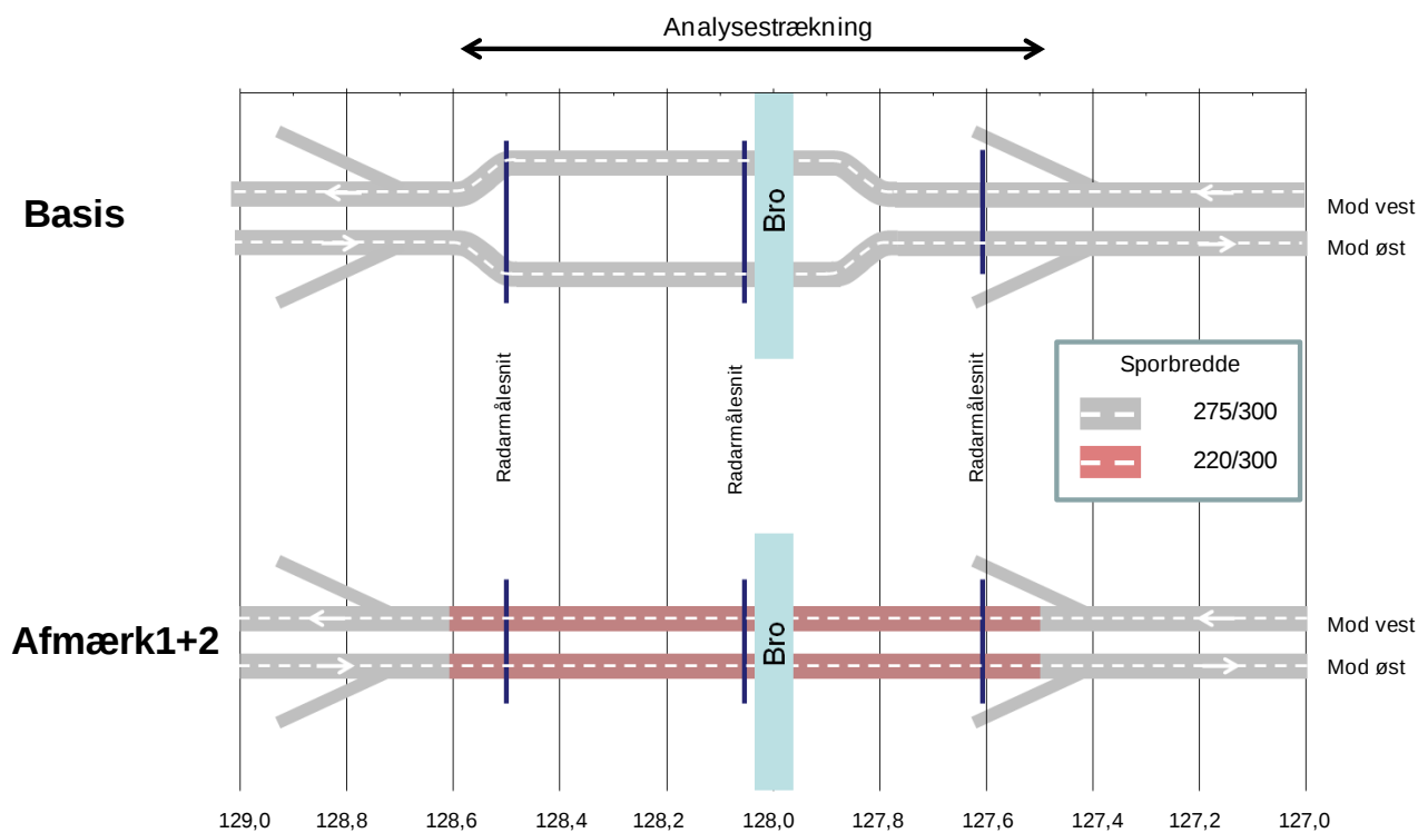
Figur 2.3. Analysestrækning i basis-situation samt ved Afmærk 1+2.
