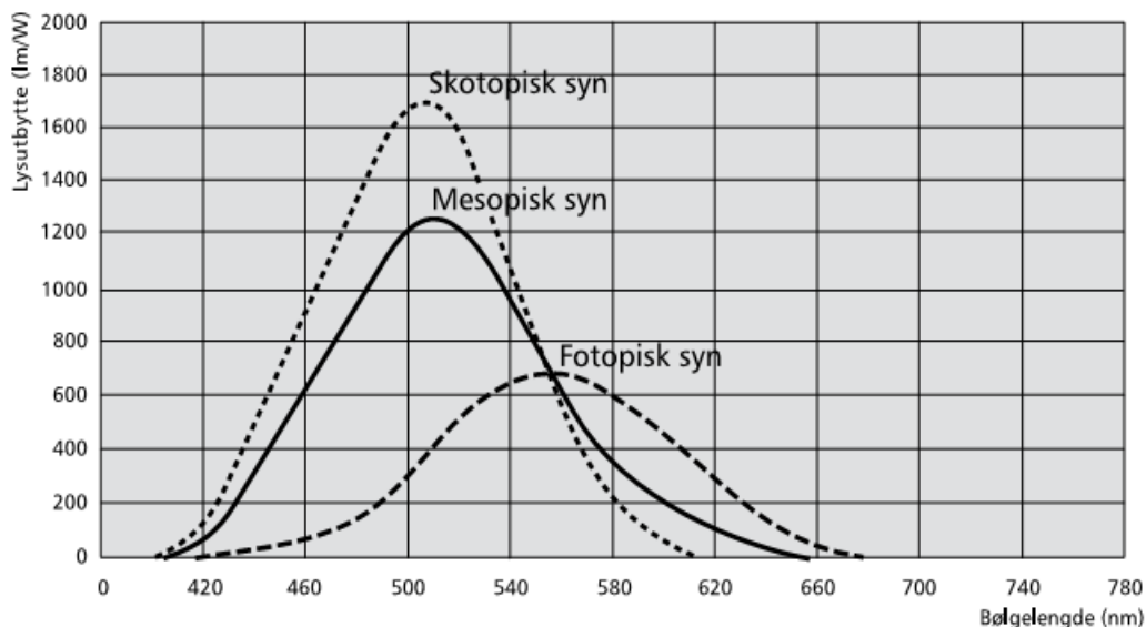
Figur 4.14: Øynenes spektrale følsomhet ved dagslys (fotopisk syn), nattlys (skotopisk syn) og kunstig belysning slik som vegbelysning (mesopisk syn)
