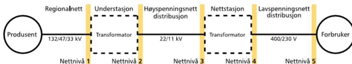
Figur 5.1: Ulike nettnivåer
