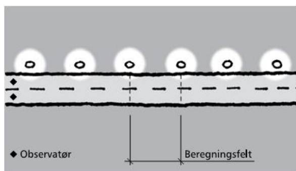
Figur 4.4: 2-felts veg, ensidig armaturrekke
