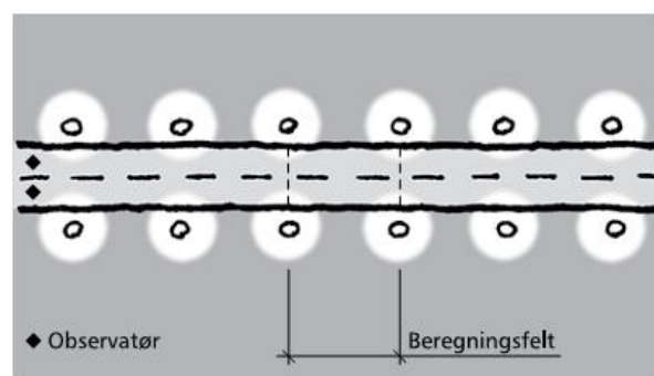
Figur 4.5: 2-felts veg, 2 armaturrekker
