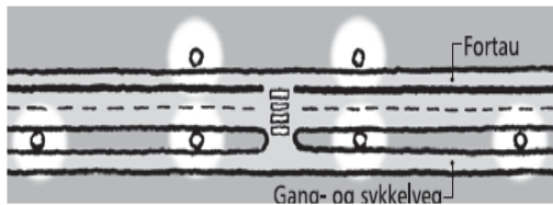
Figur 3.3: Prinsippskisse for forsterket belysning
