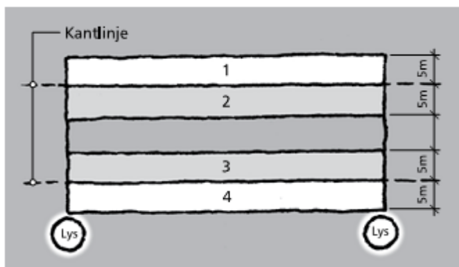
Figur V1.0.1: Omgivelsesforhold SR = (1+4)/(2+3) der tallene representerer gjennomsnittlig belysningsstyrke i hvert område. Områdebredden reduseres fra 5 m til \frac{1}{2} kjørebanelbredde når denne er smalere enn 10 m.
