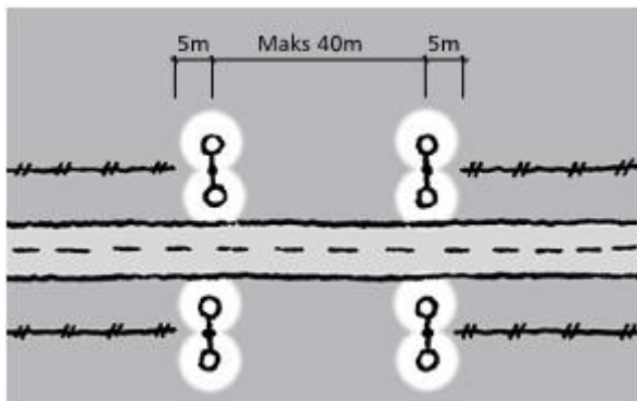
Figur 4.10: Masteplassering ved viltkryssinger
