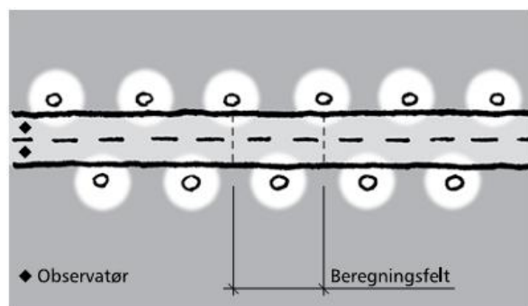
Figur 4.6: 2-felts veg, 2 armaturrekker i sikksakk
