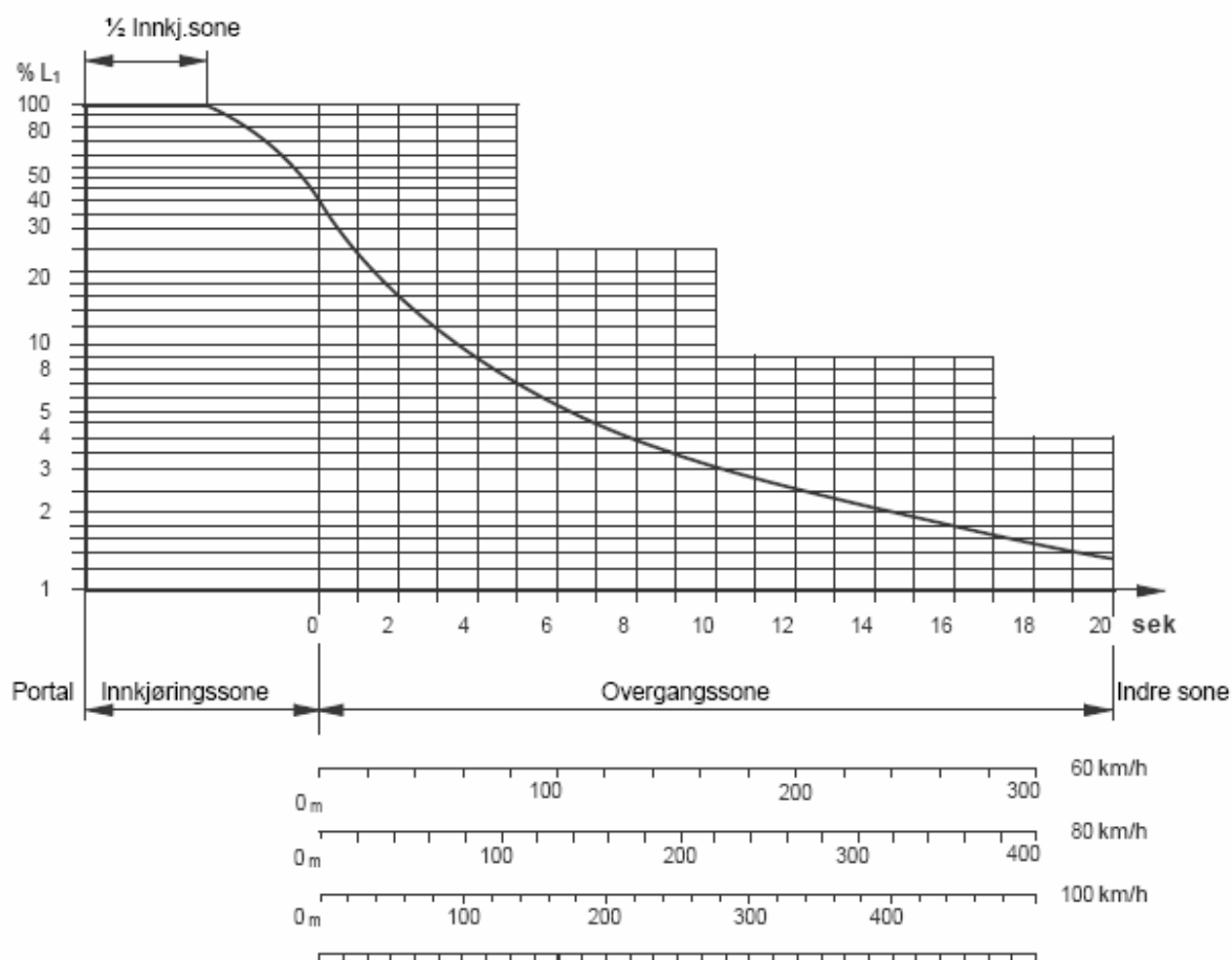
Figur 9.2: Luminansreduksjonskurve for dagslysforhold
