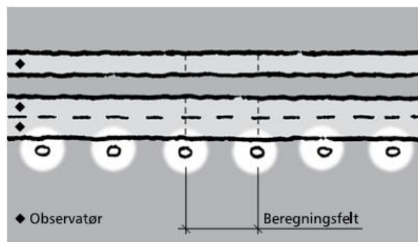
Figur 4.2: 3-felts veg med midtrabatt, ensidig armaturrekke, 2 beregningsfelt
