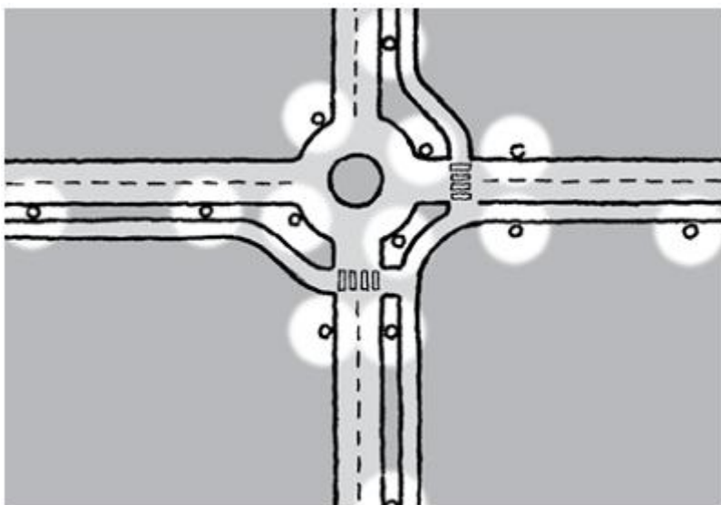
Figur 4.7: Eksempel på belysning av rundkjøring
