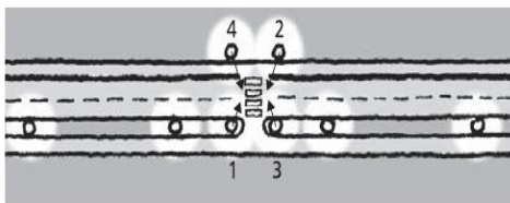
Figur 3.2: Prinsipp-skisse for intensivbelysning av gangfelt
