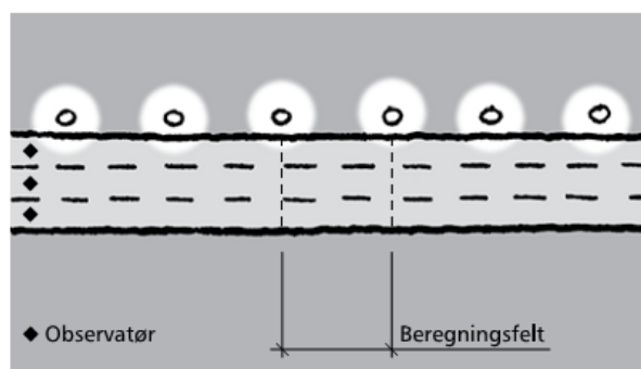
Figur 4.3: 3-felts veg, ensidig armaturrekke
