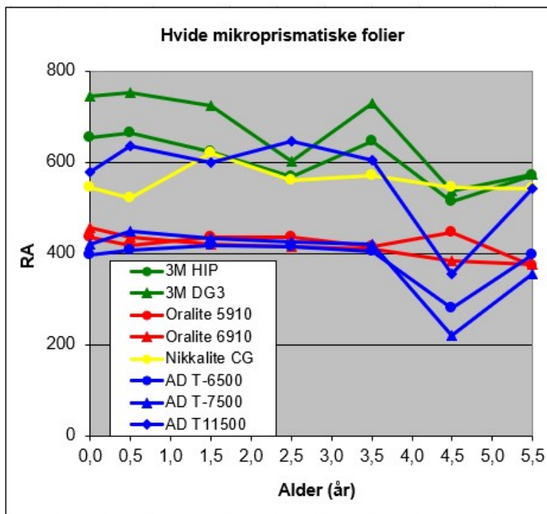
Figur 5: Forløb af R_A værdier for hvide mikroprismatiske folier.
