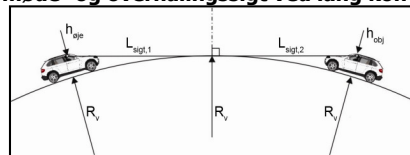
Stop-, møde- og overhalingssigt ved lang konveks kurve
