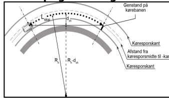
Stopsigt ved lang kurve
