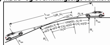
Stop-, møde- og overhalingssigt ved kort konveks kurve
