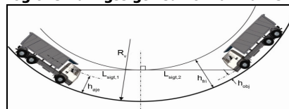
Stop-, møde- og overhalingssigt ved konkav kurve ved sigthindring
