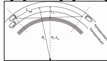
Mødesigt og overhalingssigt ved lang kurve
