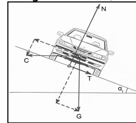
Tværfald og radius med kørselsdynamik
