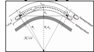
Stop-, møde- og overhalingssigt ved ko
