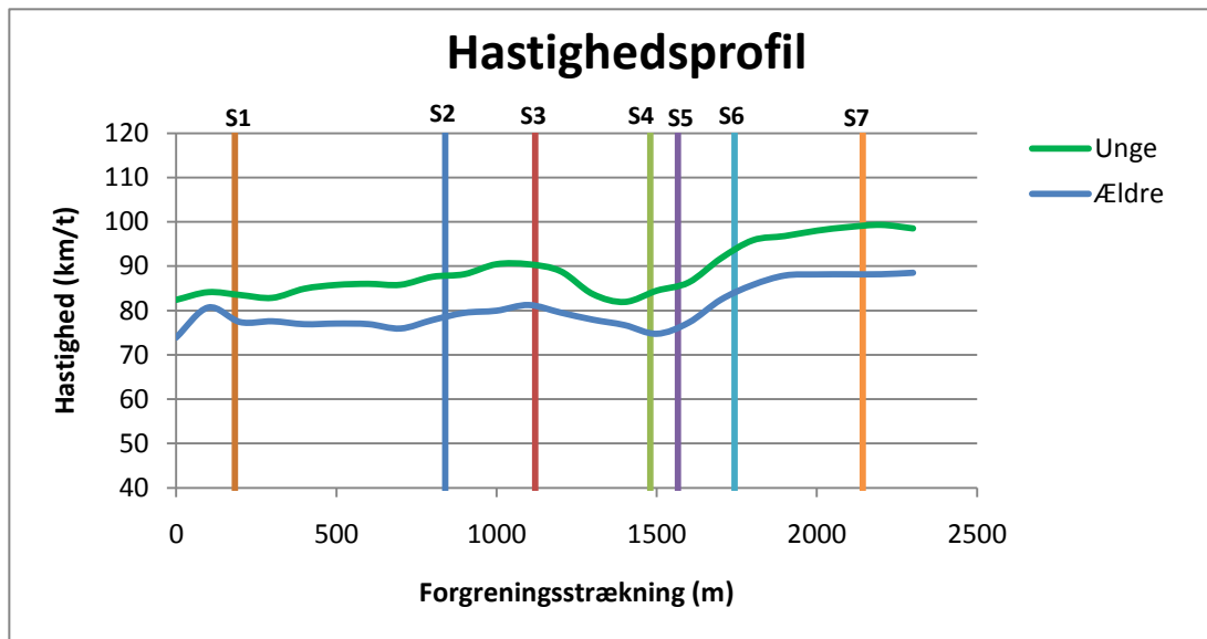
Figur 3.6. Gennemsnitligt hastighedsprofil for hhv. unge og ældre på forgretningsstrækningen. De lodrette farvemarkeringer angiver placeringen af de syv vejvisningstavler.
