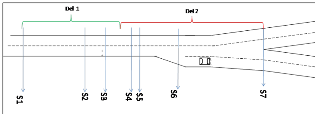
Figur 3.10. Principskitse. Ved registrering af kognitiv belastning opdeles forgreningsstrækningen i Del 1 og Del 2, hvor Del 2 ligger tættest på divergenspunktet. Længden af hver af de to delstrækninger er ca. 980 m.
