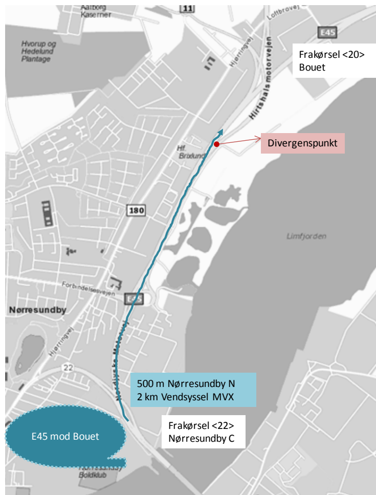
Figur 2.3 Oversigtstegning af forgreningsstrækning.
