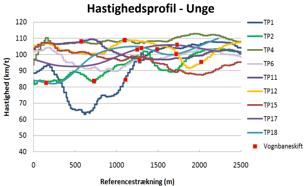
Figur 3.2. Hastighedsprofil for unge testbilister (TPX) på referencestrækning, med angivelse af hvor på strækningen vognbaneskit påbegyndes.
