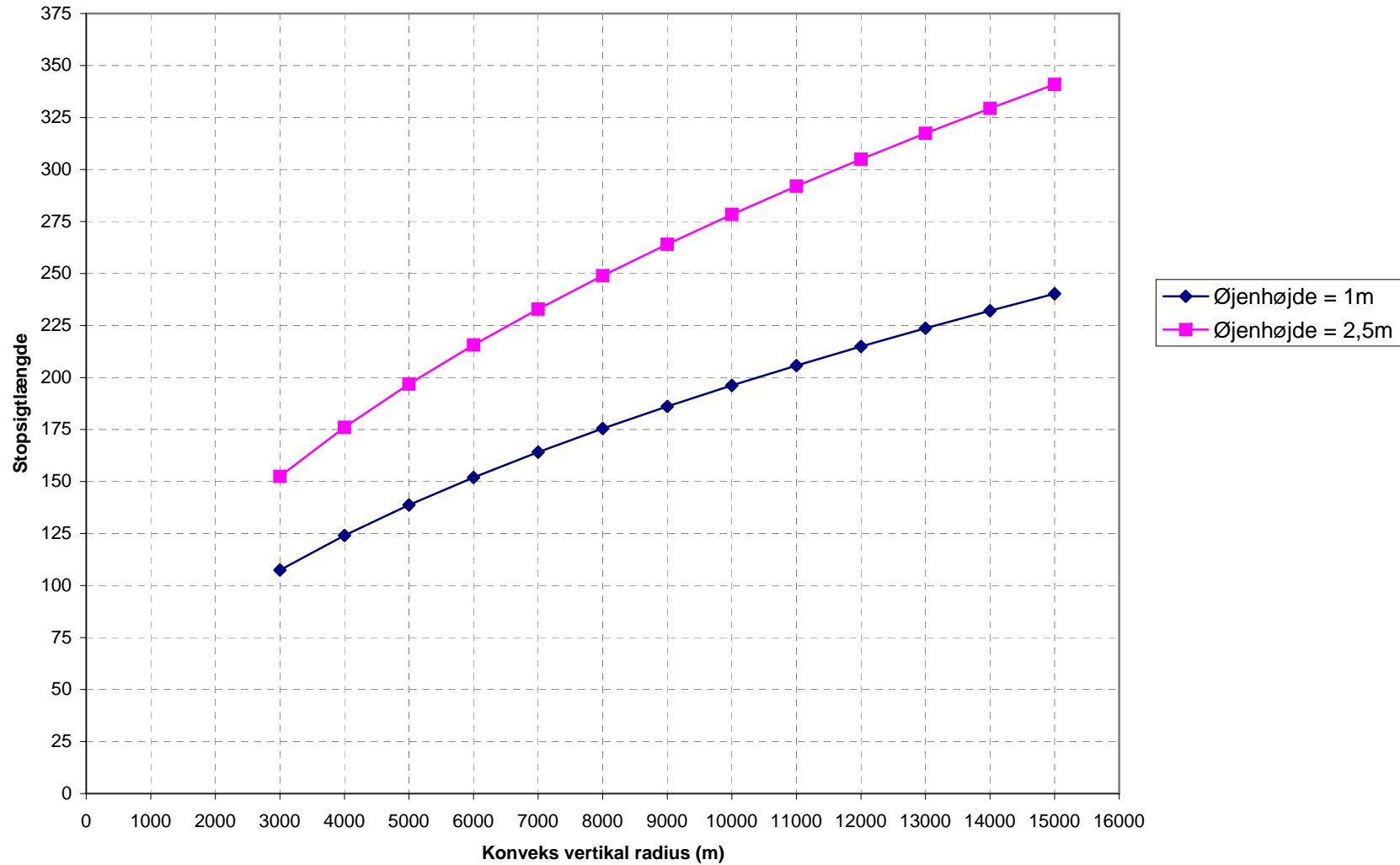
Stopsigtlængde som funktion af vertikal radius (lang kurve) for øjenhøjde 1 og 2,5m
