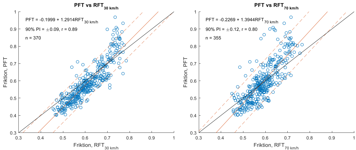
Figur 14. Jämförelse mellan PFT och RFT_{30\text{ km/h}} (vänster) samt mellan PFT och RFT_{70\text{ km/h}} (höger). Blå markeringar: observationer. Röd heldragen kurva: regressionslinje. Röd streckad kurva: prediktionsintervall. Svart kurva: y=x .
